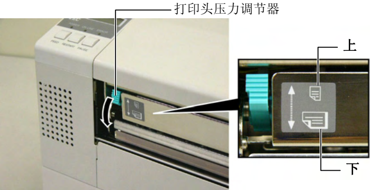
注释: 打印头压力调节器位置
